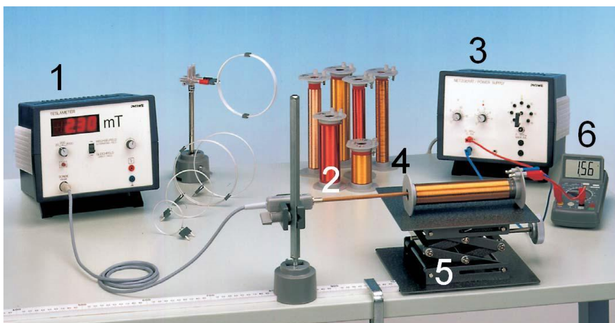
Rys.1. Zestaw pomiarowy: 1 - teslomierz, 2 - sonda Halla, 3 - zasilacz solenoidu, 4 - solenoid (cewka), 5 - podnośnik cewki, 6 - amperomierz.
